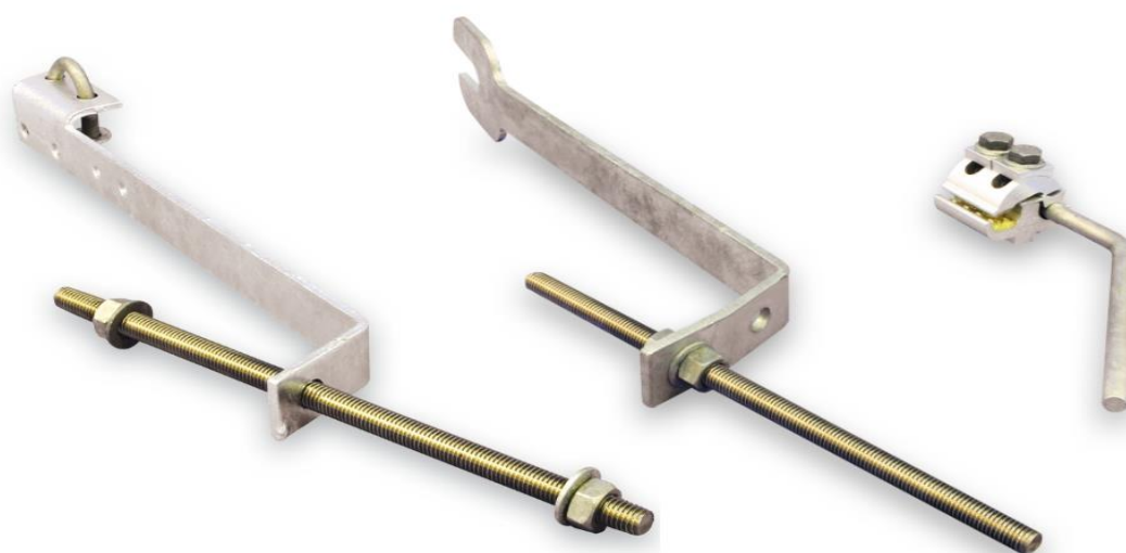
شکل ۲ - تخلیه قوس الکتریکی (مجهز به شاخک تخلیه قوس و پایه)
